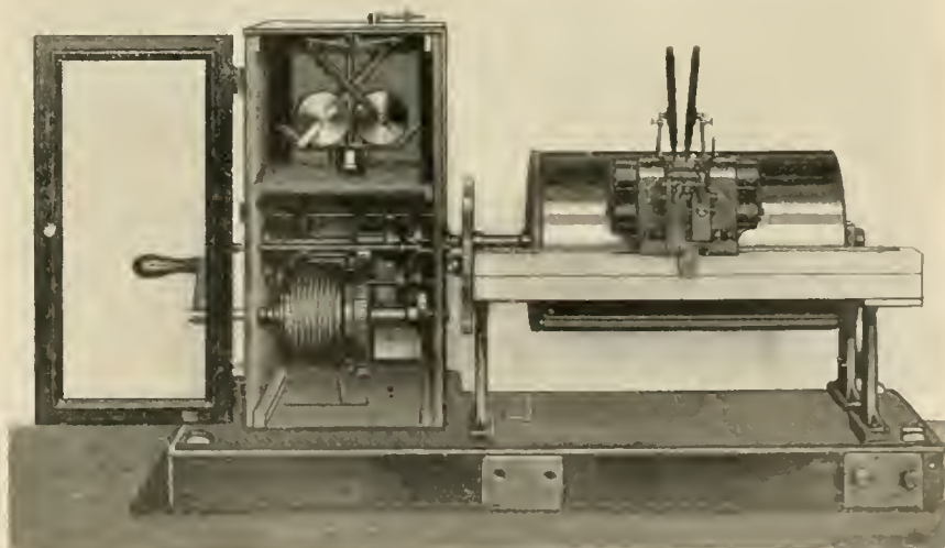
FIG. A. THE CHRONOGRAPH.
